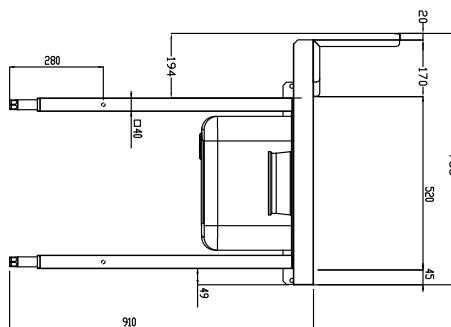
Zij aanzicht
